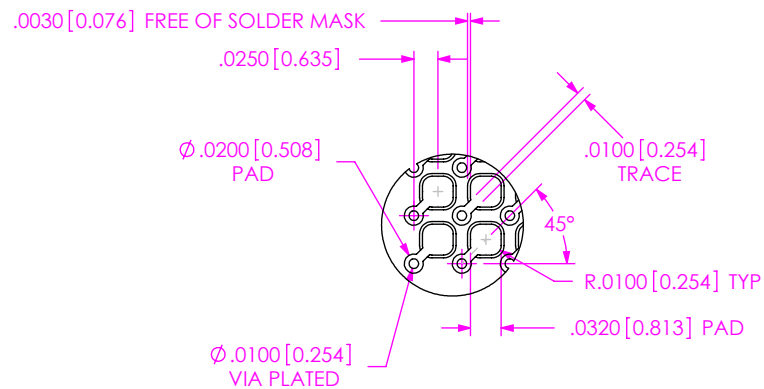
DETAIL 'B' SCALE 5:1
