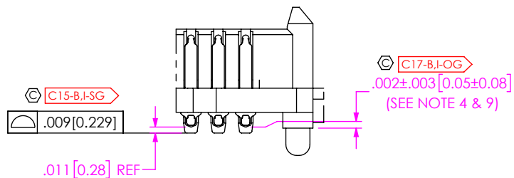
DETAIL 'B' SCALE 4 : 1
