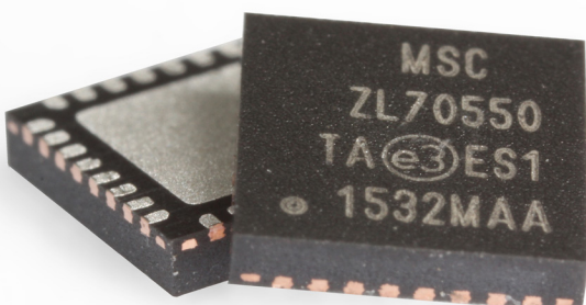
QFN package actual size: 5 mm x 5 mm
