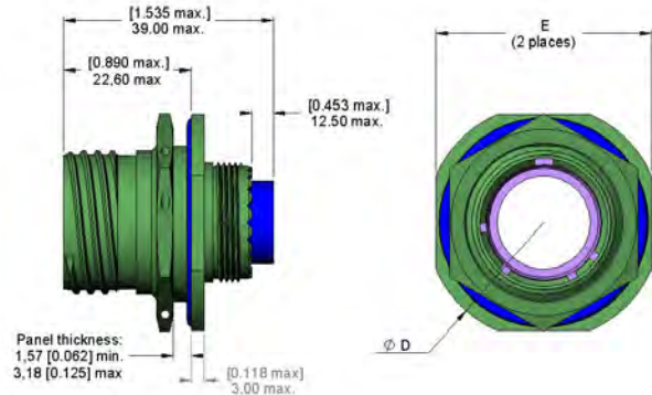
Fig. 2 Jam nut receptacles
