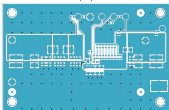
Top Layer
