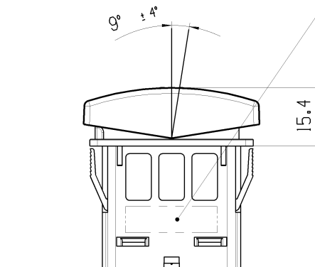
Ausführung mit Kappe B Version with cap B
