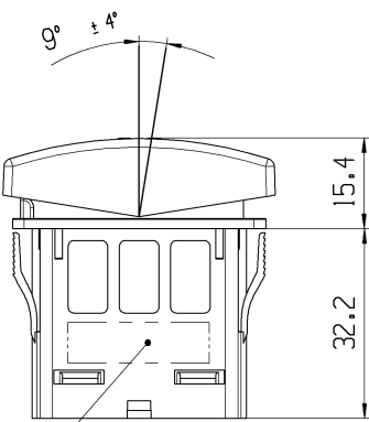
Ausführung mit Kappe B Version with cap B
