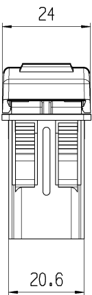
Ausführung mit Kappe A Version with cap A
