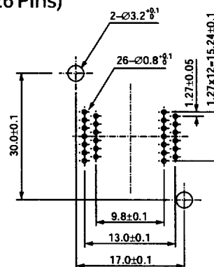
TSOP IC51-0442-1709 (44 Pins)
