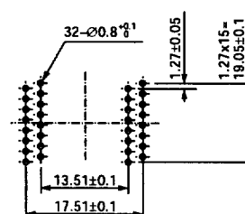
SOP IC51-0322-667-2 (32 Pins)
