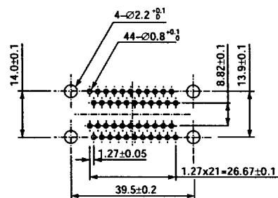
SOP IC51-0442-1208 (44 Pins)
