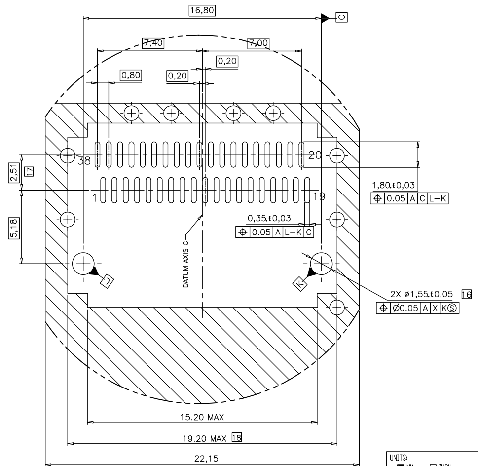
DETAIL Z 2:1
