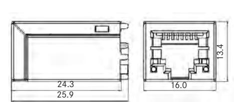
Y-ConJack-51
