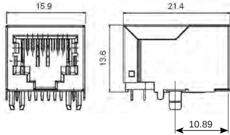
Y-ConJack-21
