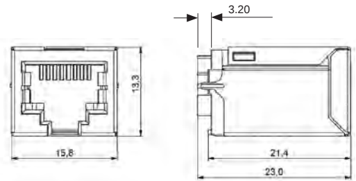
Y-ConJack-12
