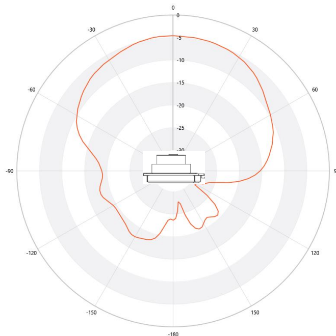
L5 RHCP Pattern @1164 MHz
