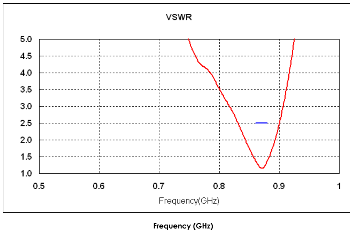
VSWR
