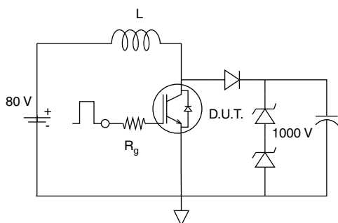
Fig. 22 - RBSOA Circuit
