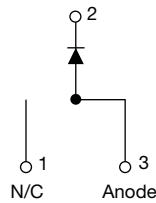
VS-8ETU04-1PbF
