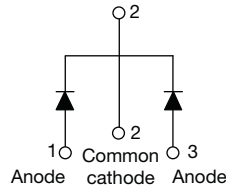
VS-48CTQ060-1PbF
