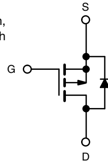
P-Channel MOSFET
