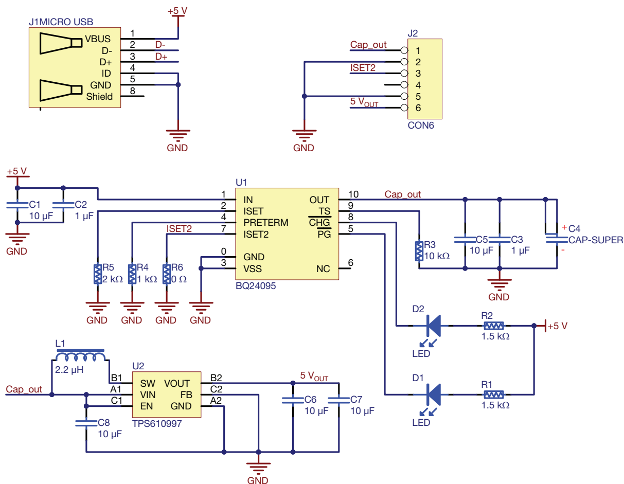
Fig. 3 - Schematic of mini charger
