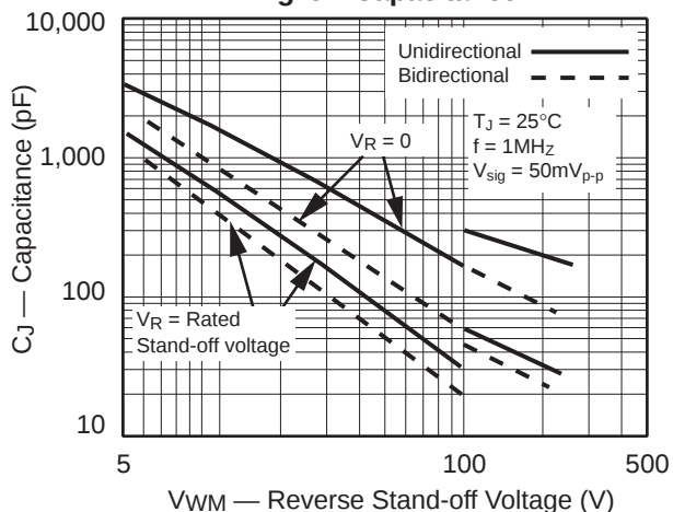
Fig. 6 – Capacitance
