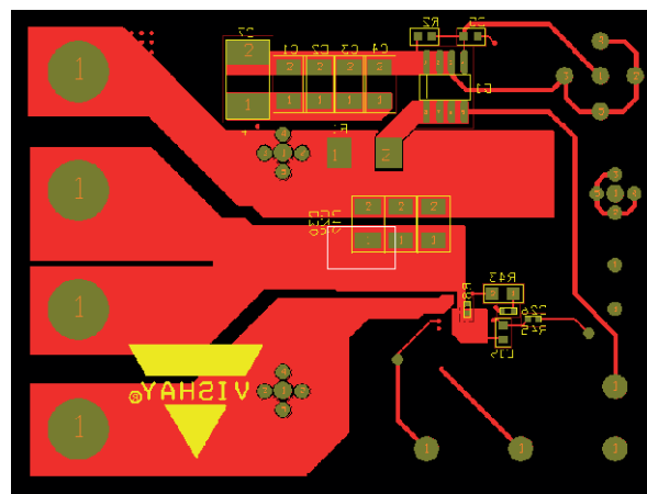
Fig. 11 - Bottom Layer
