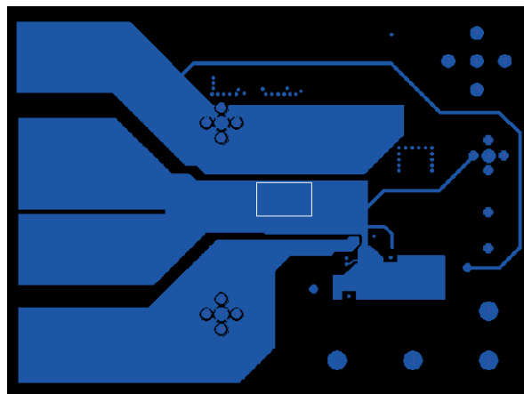
Fig. 12 - Inner Layer2
