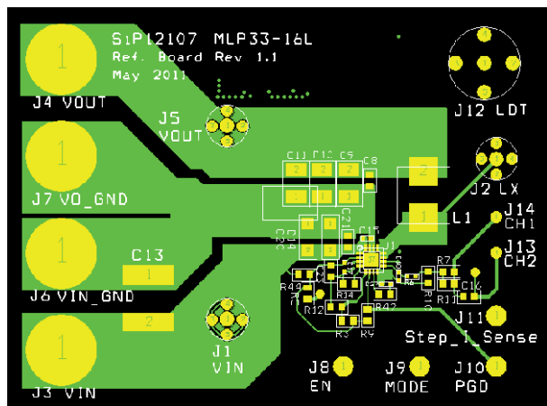
Fig. 9 - Top Layer
