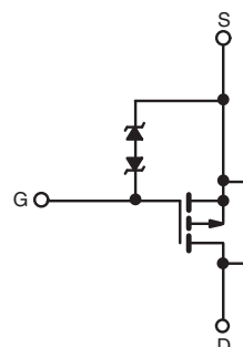
P-Channel MOSFET
