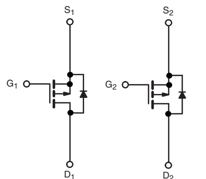
P-Channel MOSFET P-Channel MOSFET
