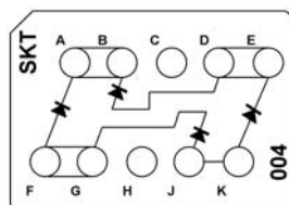
CTJ420E004 One W110 VARO Rectifier
