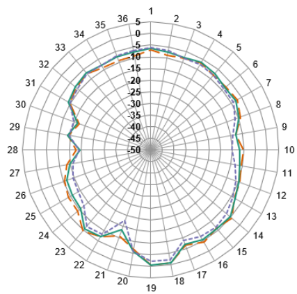
YZ-Plane Gain
