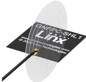
YZ-Plane Gain
