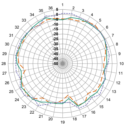
YZ-Plane Gain
