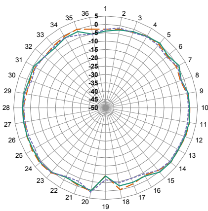
YZ-Plane Gain
