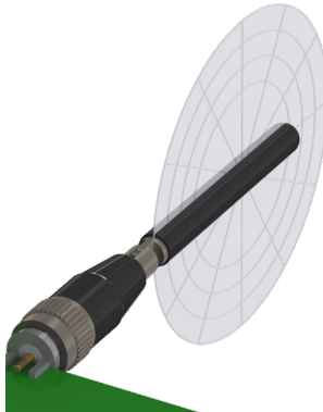
YZ-Plane Gain
