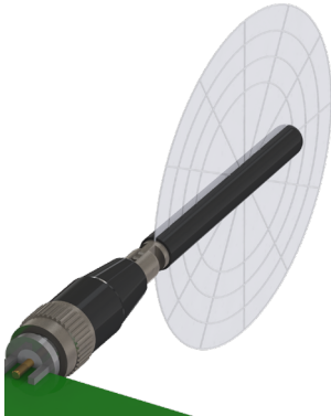
YZ-Plane Gain
