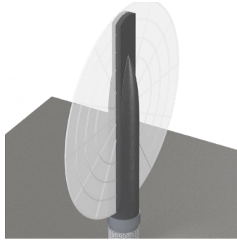
YZ-Plane Gain
