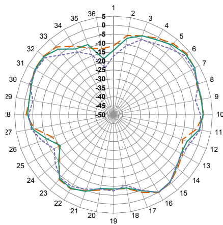
XZ-Plane Gain
