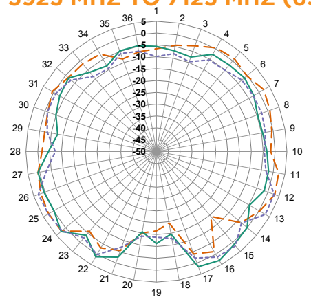
XZ-Plane Gain
