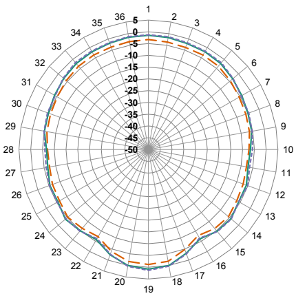
YZ-Plane Gain
