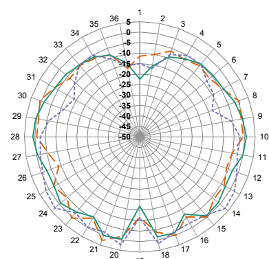
XZ-Plane Gain
