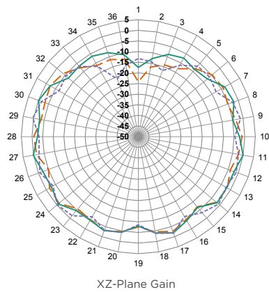
XZ-Plane Gain
