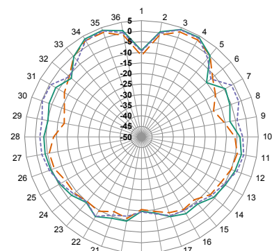
XZ-Plane Gain
