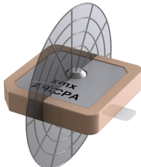
YZ-Plane Gain
