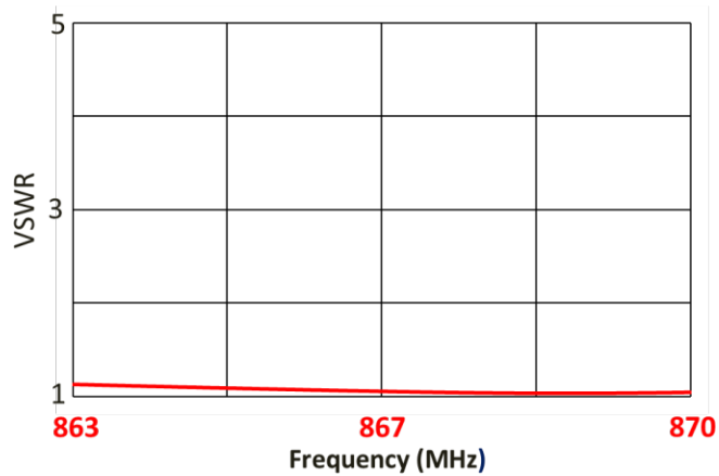
VSWR
