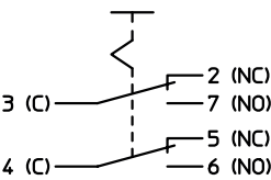
2 NO/NC Change-over
