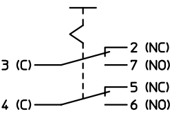
2 NO/NC Change-over
