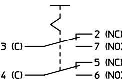
2 NO/NC Change-over
