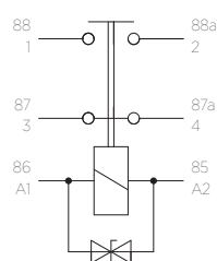
NO/NC-Contact
