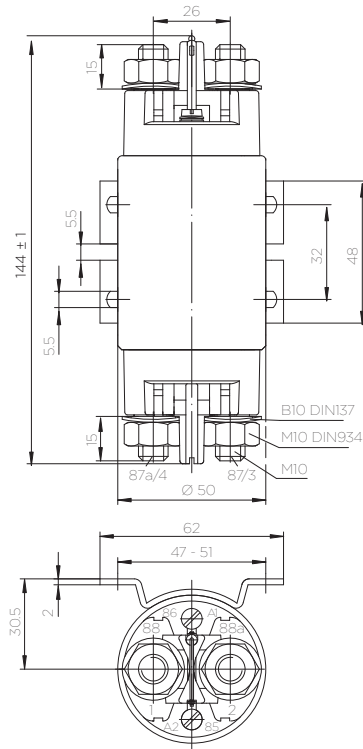
Change-over NO/NC
