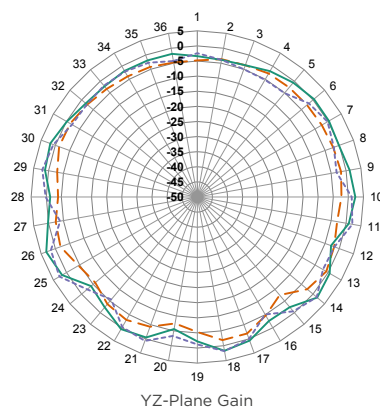
YZ-Plane Gain
