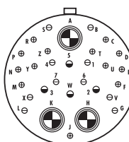
24-20 10#20 13#16 4#12 3 TWINAX #8 (N)
