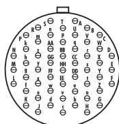
22-53 53#20 (I)
