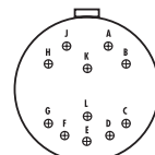
18-11 11#16 (II)
