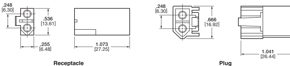
Receptacle
