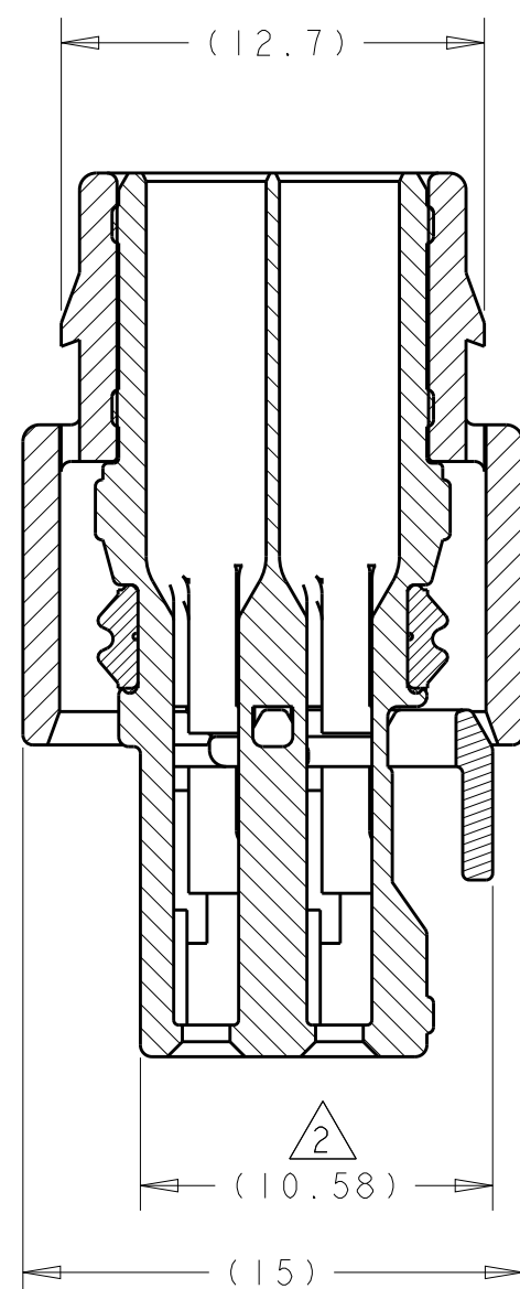
SECTION A-A
