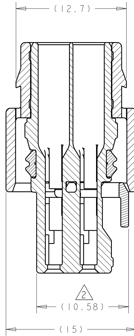
SECTION A-A
