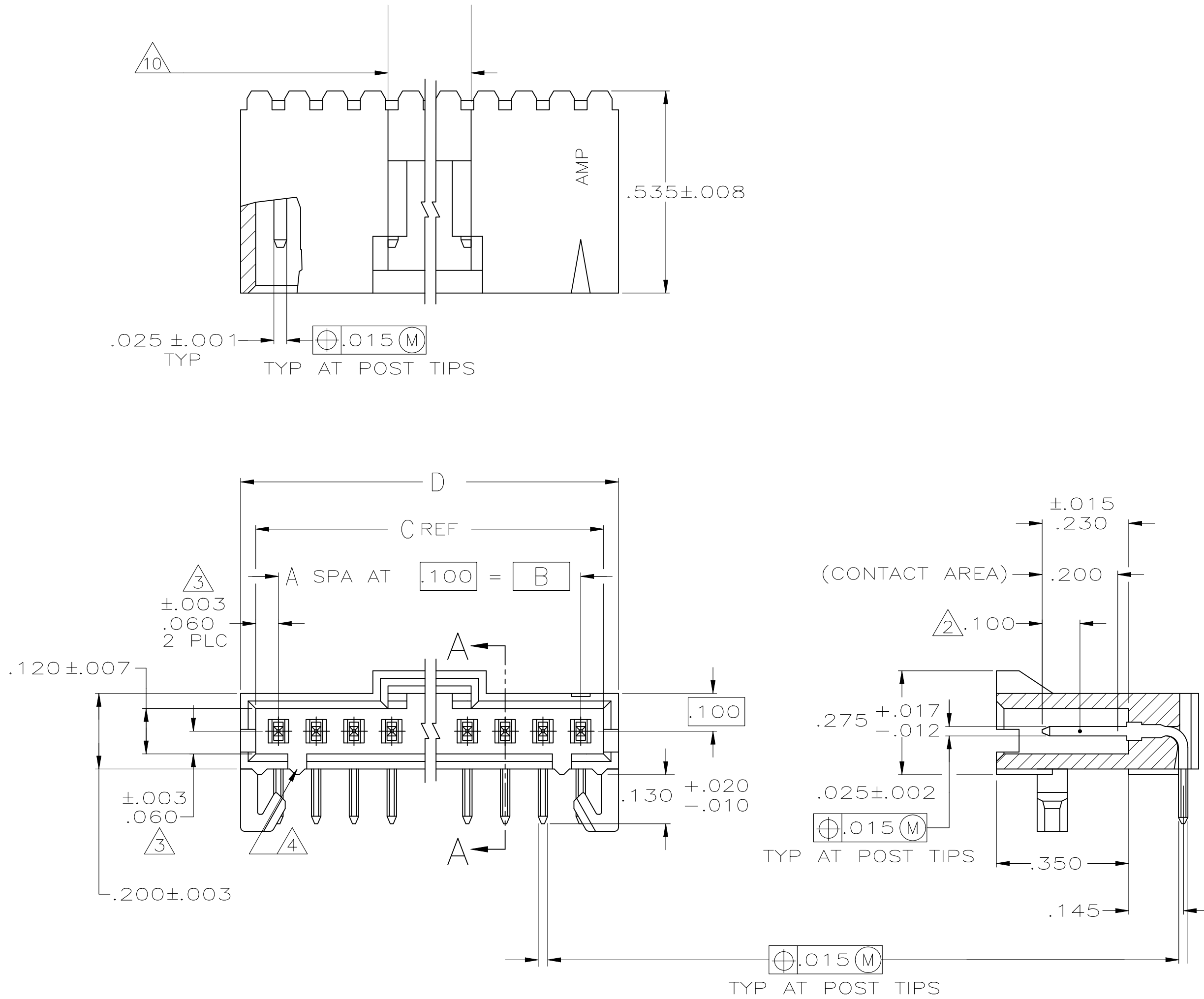
SECTION A-A
