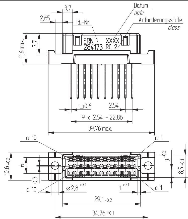
Bestückungsplan / contact layout ■ bestückt / assemble
