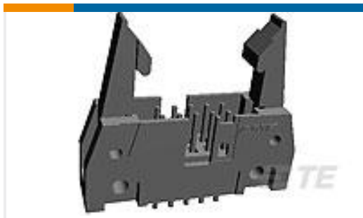
TE Part #2-5499206-8 A/L UNIV HDR 34P VERT LG LAT B
