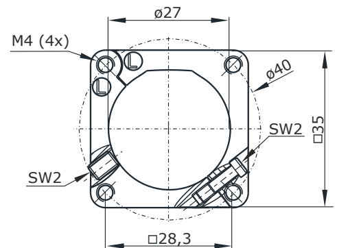
Hauptabmessungen Flansch
