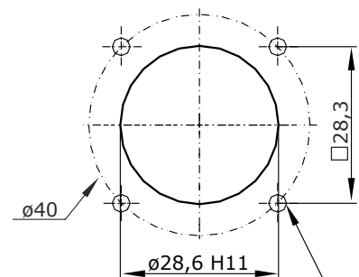
Hauptabmessungen Flansch
