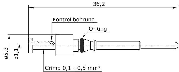
Hauptabmessungen Kontaktstift
