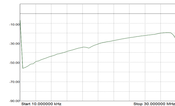
120A
