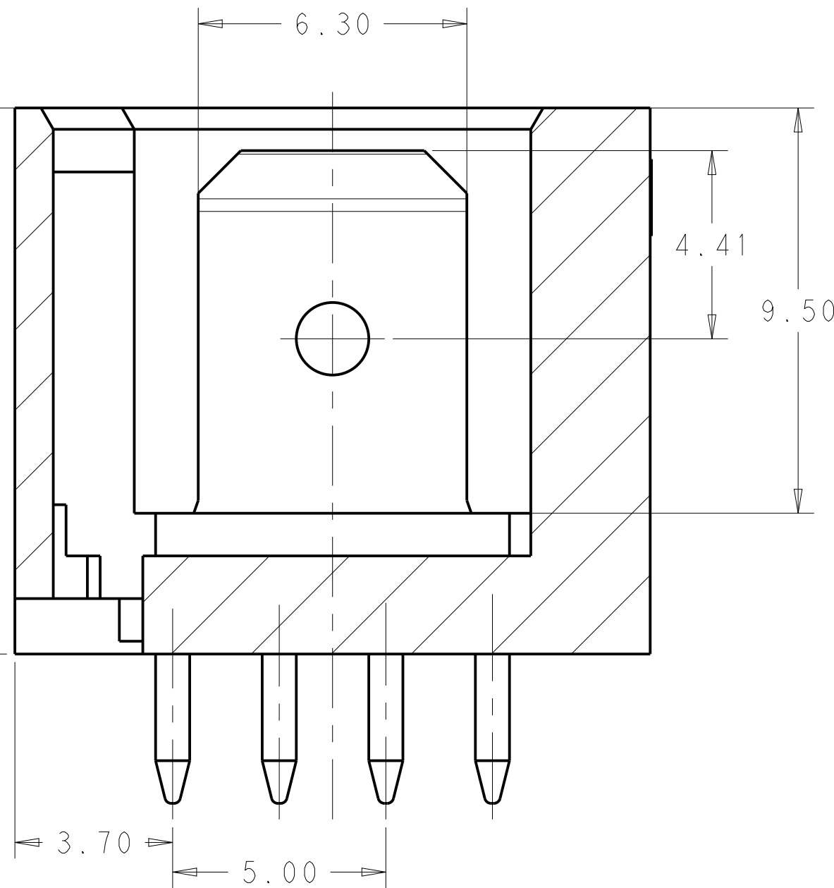
SECTION A-A
