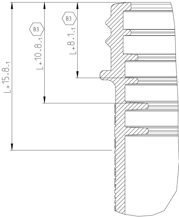
SECTION A-A Schnitt SCALE 5:1 Maßstab
